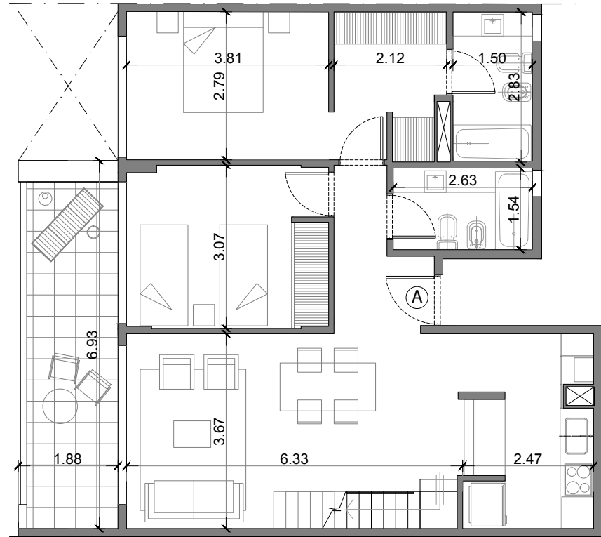
TERCER PISO
