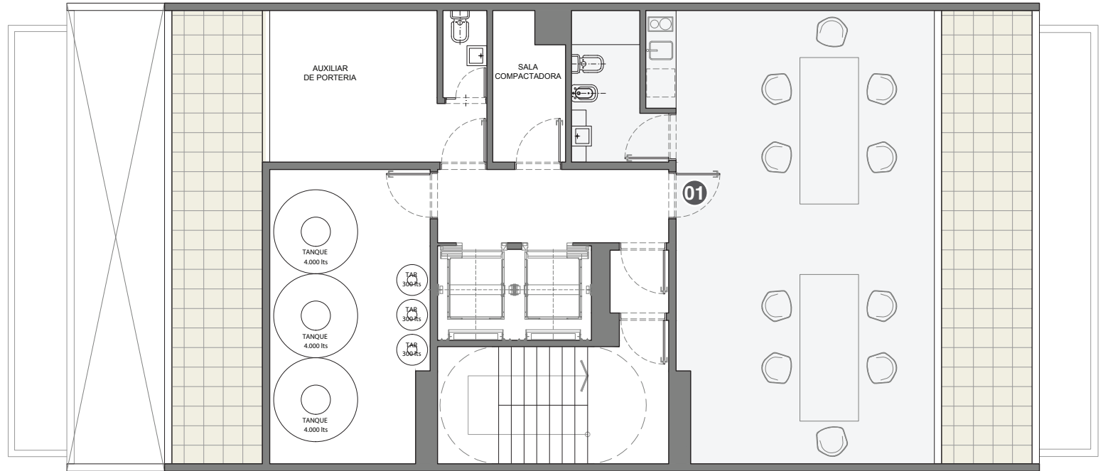
PLANTA 10° PISO
